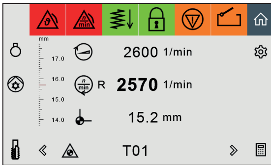
Display Hauptbildschirm
